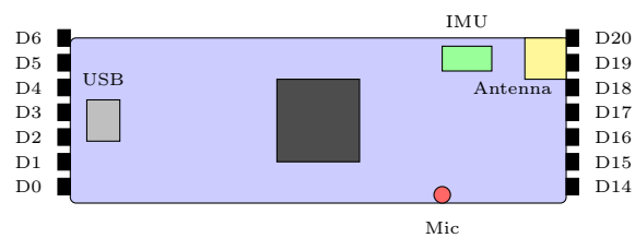
Abbildung 3.2: Arduino Nano 33 BLE Sense Lite
